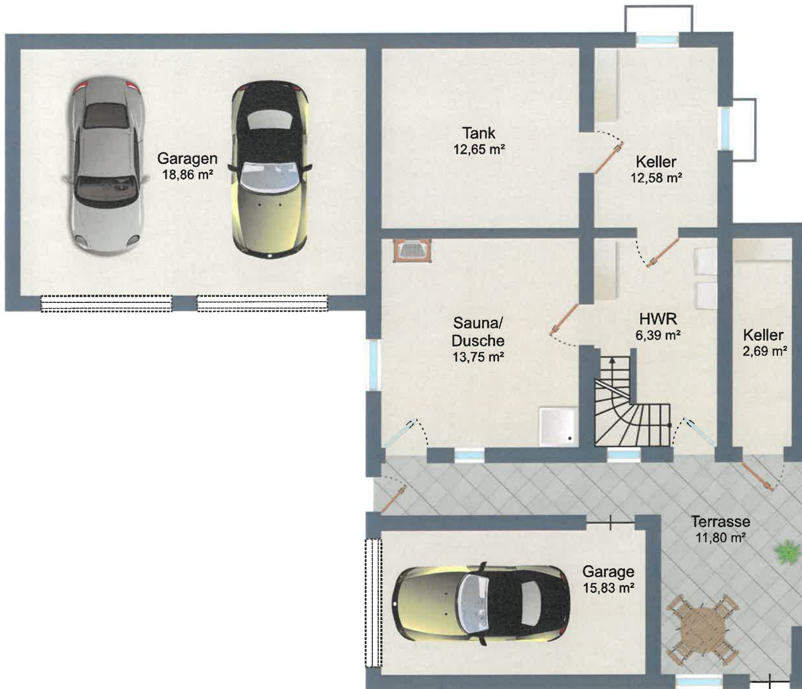
Kellergeschoss
