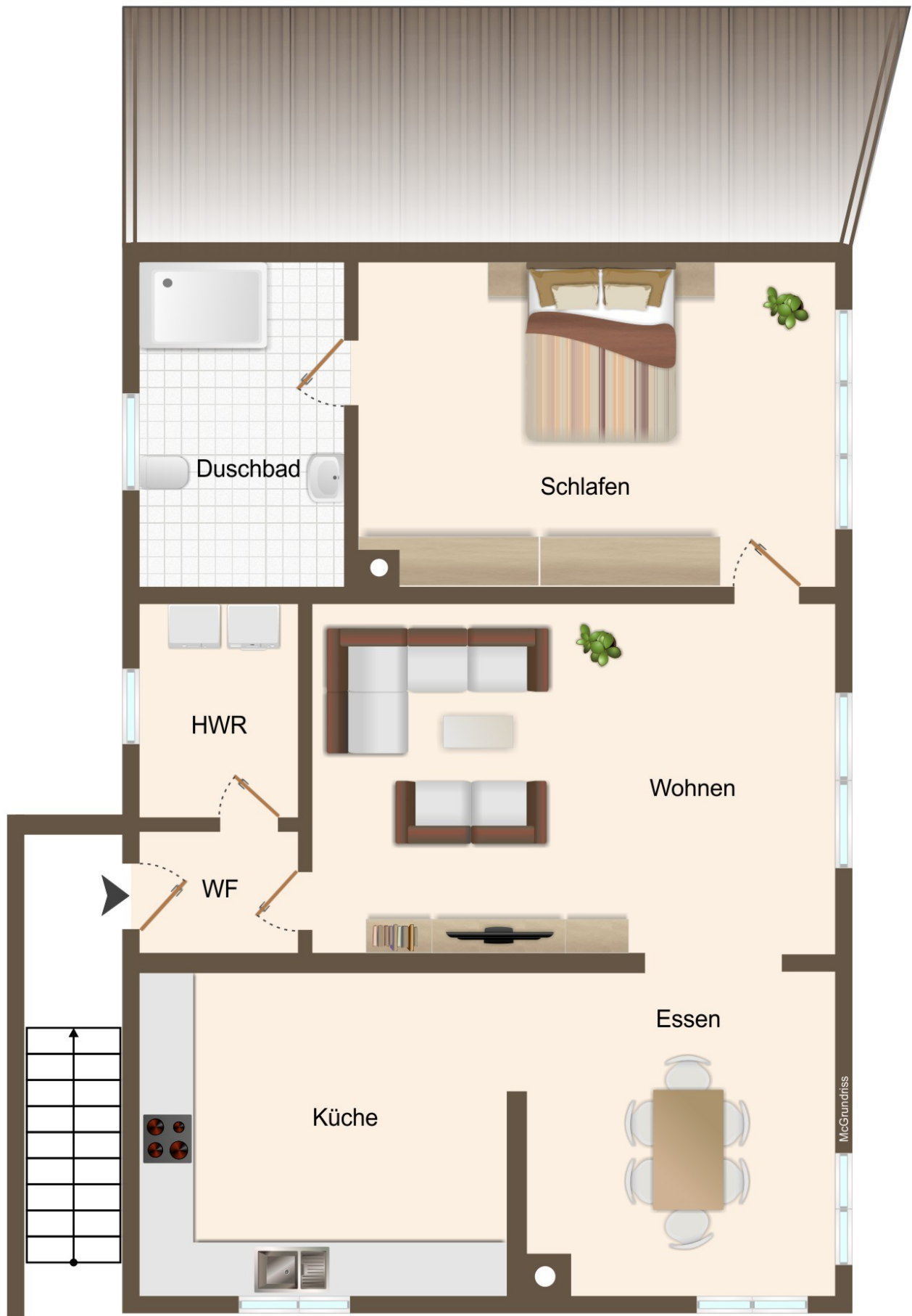
Obergeschoss Gebäude 1
